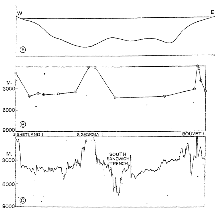
चित्र ६८—अटलांटिक महासागर के आरपार अनुप्रस्थ काट
